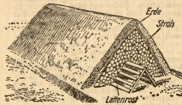
Abbildung 1. Querschnitt durch eine Kartoffelmiete mit glattem Rost zur Bodenlüftung.
