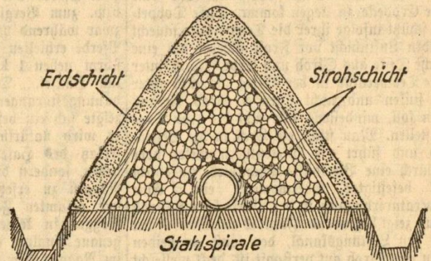
Abbildung 3. Querschnitt durch eine Kartoffelmiete mit Stahlschraube zur Bodenlüftung.
