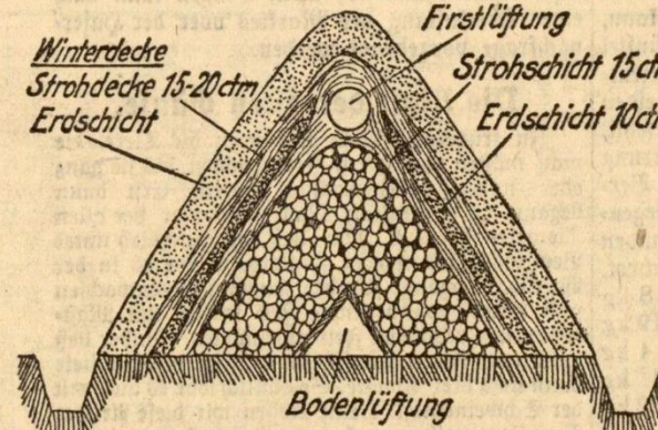
Abbildung 2. Querschnitt durch eine Kartoffelmiete mit glattem Rost zur Boden- und Firkilung.
