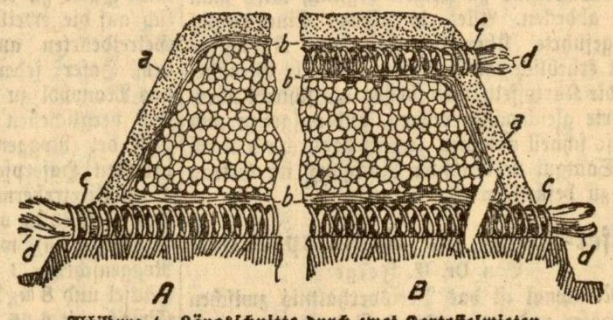
Abbildung 4. Längsschnitte durch zwei Kartoffelmieten. A mit Boden- und Firkilung, B mit Strohschicht und Firkilung.
