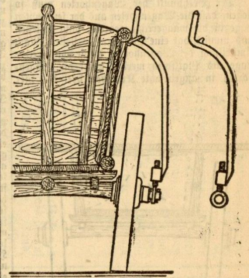
Abbildung 3. Verstellbare Stützleiste.
