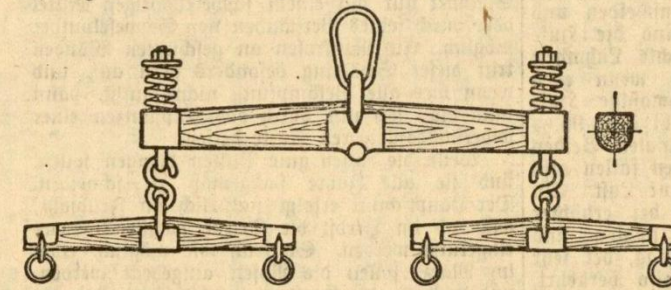
Abbildung 1. Neue Zugvorrichtung mit Holzschwengeln.
