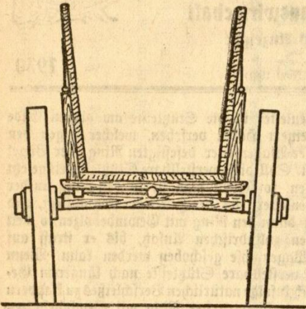
Abbildung 4. Kombiniertes Kastenwagen.
