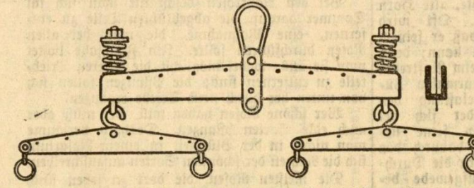
Abbildung 2. Neue Zugvorrichtung mit Eisenchwengeln.
