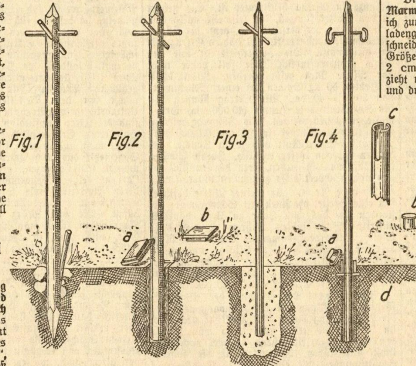
Wäsepfähle, wie sie nicht sein sollen (Fig. 1 u. 3) und wie sie zu empfehlen sind (Fig. 2 u. 4).
