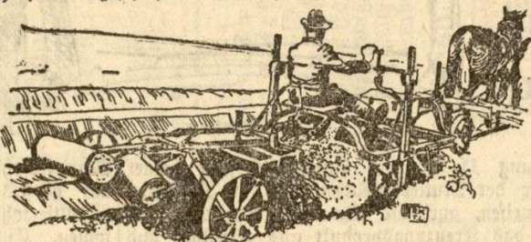
Abbildung 2. Verbesserter Zweischarhäufelpflug mit Anhänger, gerät zur Erzielung stechfertiger Beete in einem Arbeitsgang.
