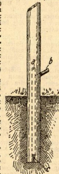
Querschnitt eines imprägnierten Zaunpfostens. a Füllröhre, b Holzpfropfen mit Sandgriff, c Holzpfropfen am Fußpunkt des Zaunpfostens.
