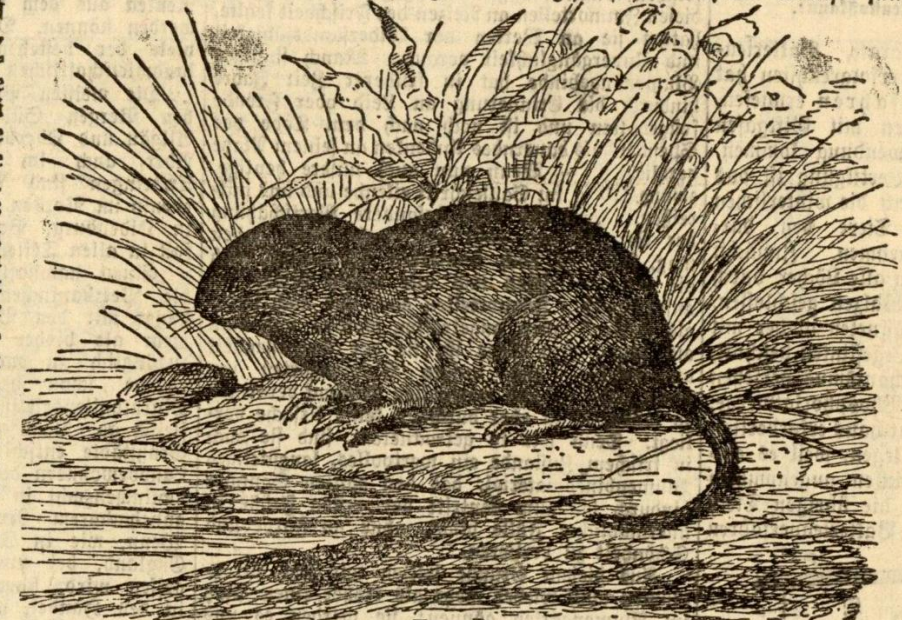
Abbildung 1. Wühlmaus.
