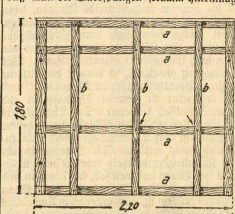
Abbildung 3. Längsseitenteil der zusammenlegbaren Gartenlaube.
