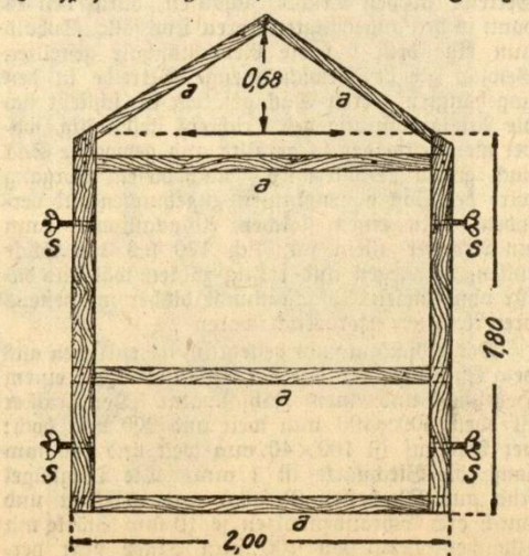
Abbildung 2. Giebel mit Querseitenteil der zusammenlegbaren Gartenlaube.
