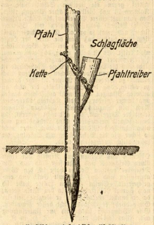
Profilierter und handlicher Pfahlreiber.
