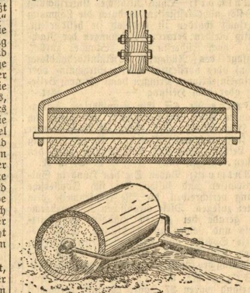
Praktische Gartenwalze.
