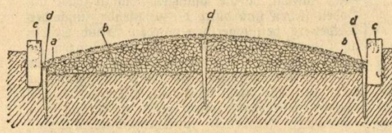
Abbildung 1. Querschnitt eines Gartenweges. a) Kiesstreue, b) Stein- oder Schlackenschüttung, c) Rantensteine, d) Markierungspfähle.
