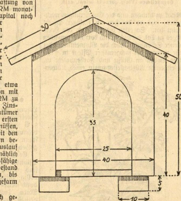
Abbildung 2. Hundehütte. Ansicht von vorn (Konstruktionszeichnung).
