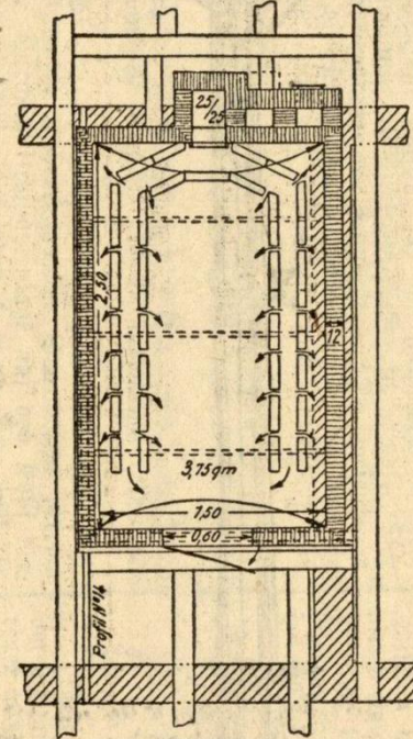
Abbildung 1. Räucherfammer im Dachboden (Grundriss).
