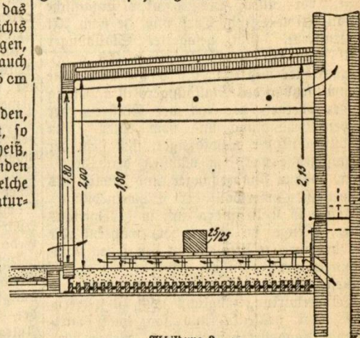
Abbildung 3. Räucherfammer im Dachboden (Querschnitt).
