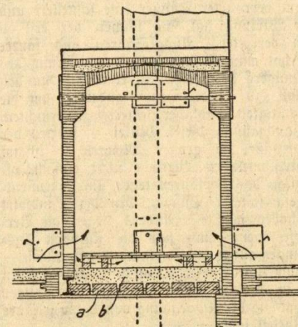
Abbildung 2. Räucherfammer im Dachboden (Querschnitt).
