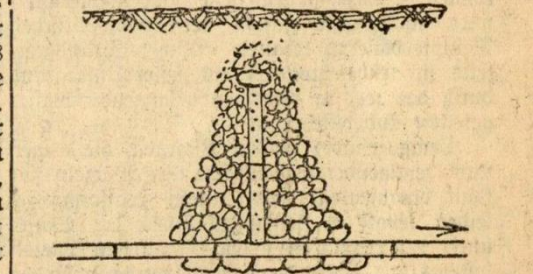
Abbildung 6. Duckentfassung durch Steinfelsen und Lochröhren.
