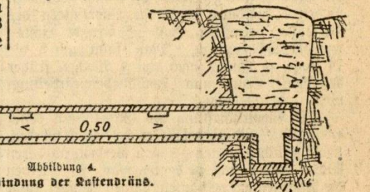
Abbildung 4. Verbindung der Rastdränung.
