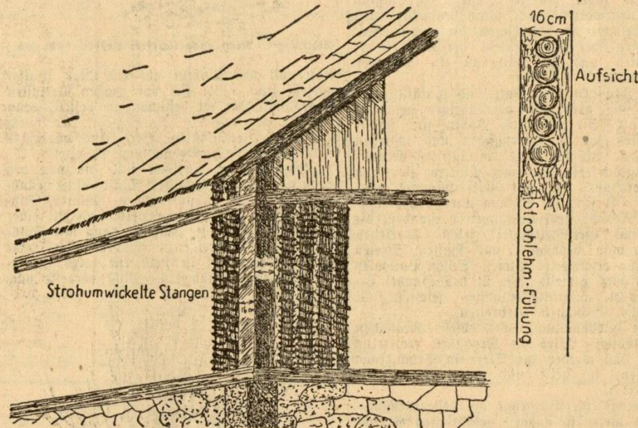
Bau der Seitenwände eines Schweinestalles.
