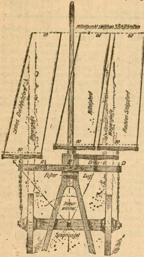
Abbildung 4. Verwirklichte, unpraktische Anspannung.
