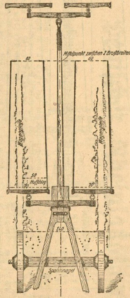
Abbildung 2. Symmetrische Anspannung für 2 und 4 Pferde.
