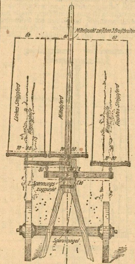
Abbildung 5. Annähernde Anspannung, aber symmetrisch richtig.
