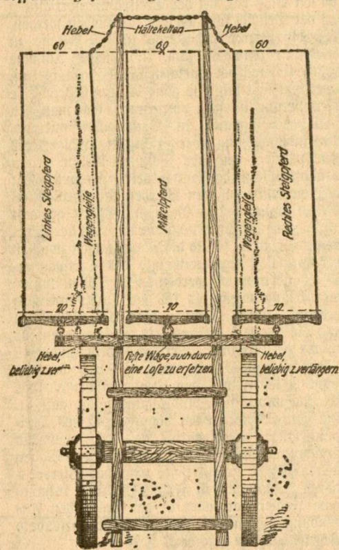
Abbildung 1. Symmetrische Anspannung für 3 Pferde mit 3 Karrenbäumen ohne Deichsel.
