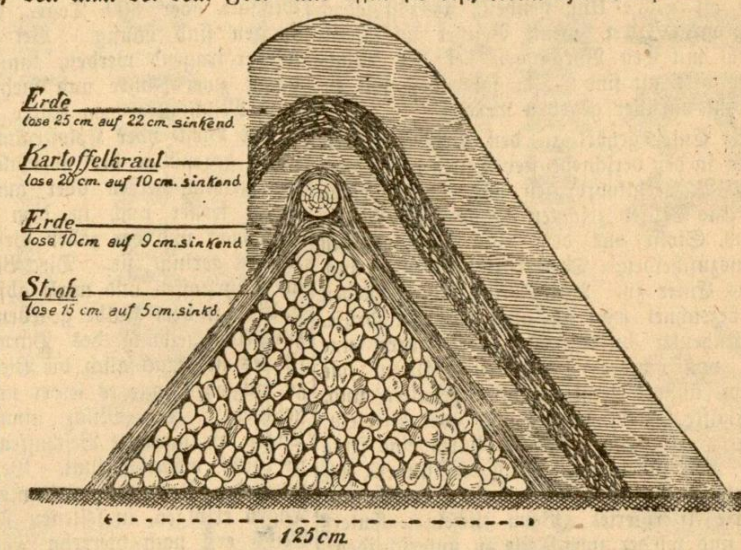
Abbildung 3. Kartoffelmiete mit Winterdede.
