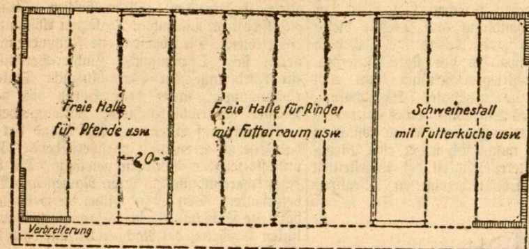
Abb. 1. Grundriss.
