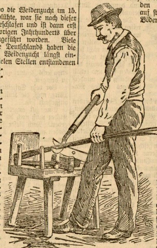
Abbildung 1. Weidenpflanzmaschine.
