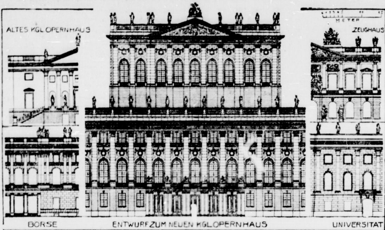
Die Größe des neuen Berliner Opernhauses am Königsplatz.
