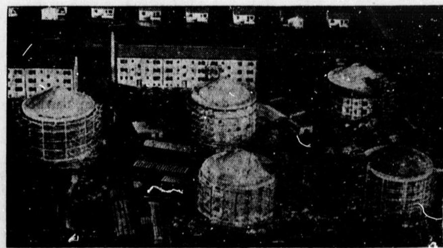
Häuser, die in einem Stockholmer Vorort errichtet werden. Die drei- bis vierstöckigen Rundbauten enthalten je Stockwerk zehn Einzelzimmer-Wohnungen, die für das Personal eines nahegelegenen Krankenhauses vorgesehen sind. Die Wohnungen sind fächerförmig um das kreisrunde Treppenhaus in der Mitte angeordnet. Die Häuser werden in verschiedenen Farbtönen getüncht.
