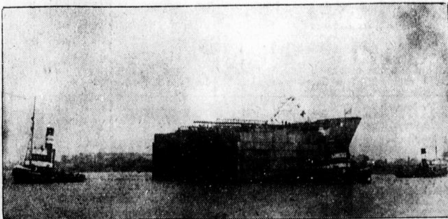
Tanker-Vorschiff vom Stapel
