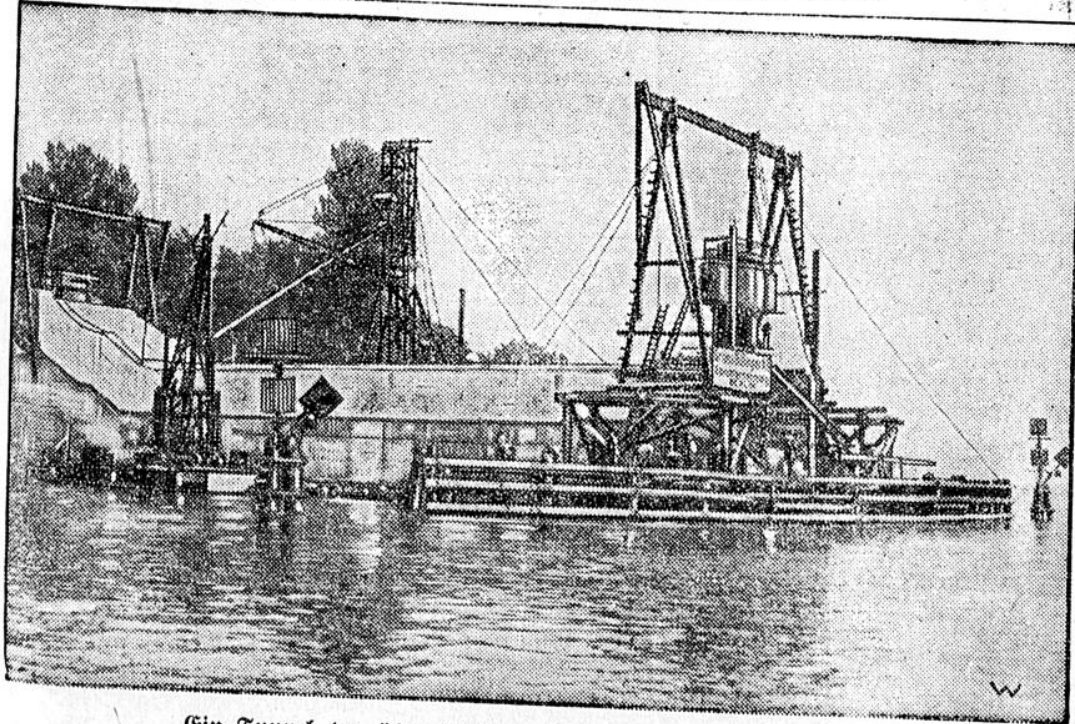
Ein Tunnel, der über Wasser gebaut und dann versenkt wird.
