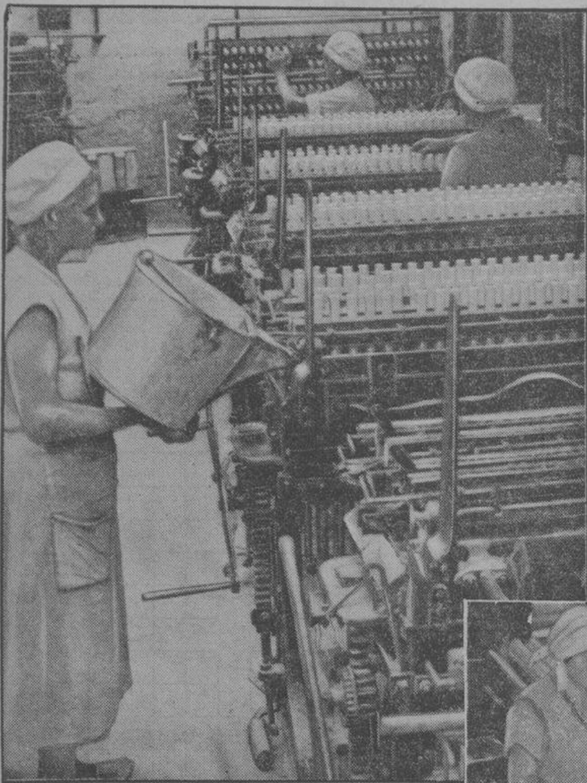
In die Gießmaschine wird das dickflüssige Stearin eingegossen und läuft in die Formen.
