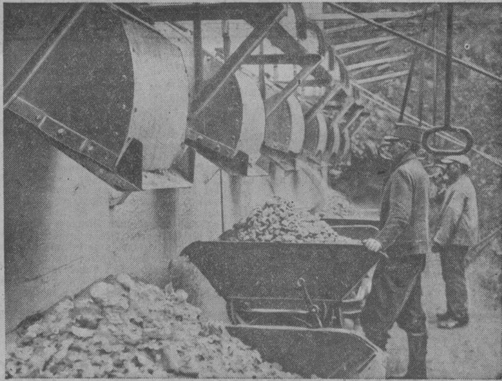
Die rohen Brocken des goldhaltigen Erzes werden zerkleinert und kommen dann zur Aufbereitung in die großen Waschanlagen.
