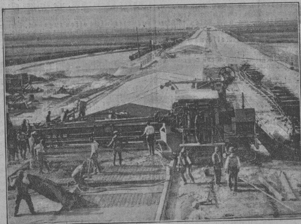
Beginn der Betonierungsarbeiten auf der Straße München – Holzkirchen. Interessant ist hier die Großzügigkeit, mit der die Bauten durchgeführt werden. Im Vordergrund sieht man die eigenartige Betonierungsmaschine. Die schrägen Dächer links sollen eine allzu rasche Austrocknung verhindern, ebenso wie die Tücher, die die Arbeiter über die untere Betondecke legen.
