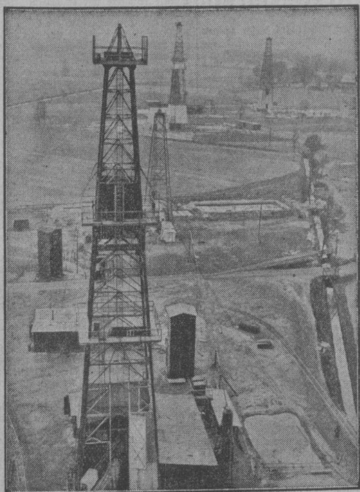
Bild vom Bohrturm der Refordquelle bei Nienhagen.
