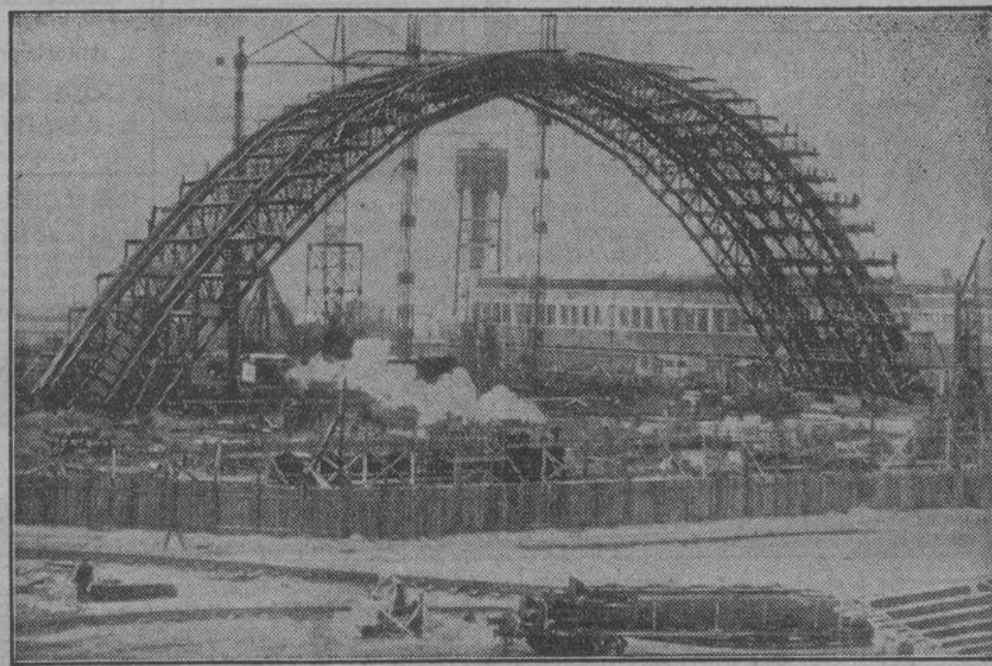
Auf dem riesigen Ausstellungsgelände vor den Toren Brüssels ist die Arbeit zum Aufbau der 1936 dort stattfindenden Weltausstellung in vollem Gange. Unser Bild zeigt das Gerüst für den riesigen Ausstellungseingangsbogen und (rechts) den gewaltigen Festpalast im Bau.
