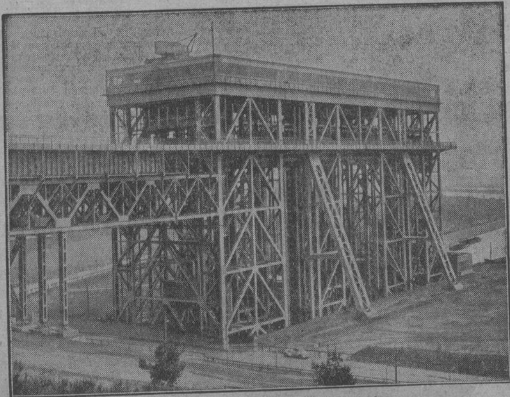
Der gewaltige Bau des Schiffshebewerks.
