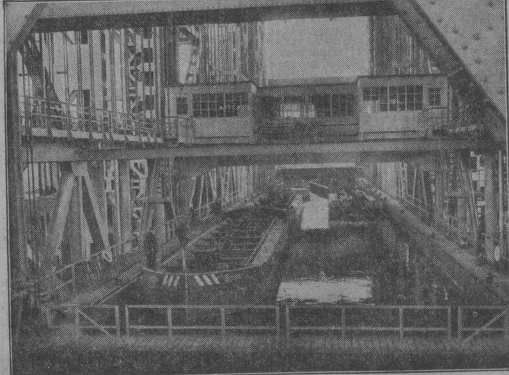
Der riesige fahrradähnliche Trog.
