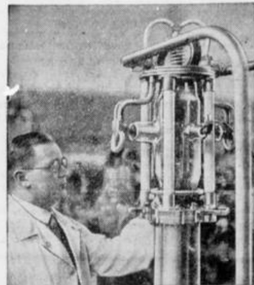
300.000 Watt aus einer Röhre. Die Telefunken-Senderöhren von 300 kW-Spannung arbeiten heute in allen deutschen Großsendern.
