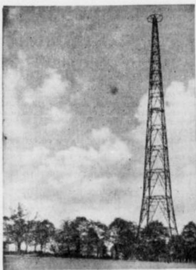
Die Ginturm-Antenne des neuen Mittelwellensenders Langenberg. Im Hintergrund
