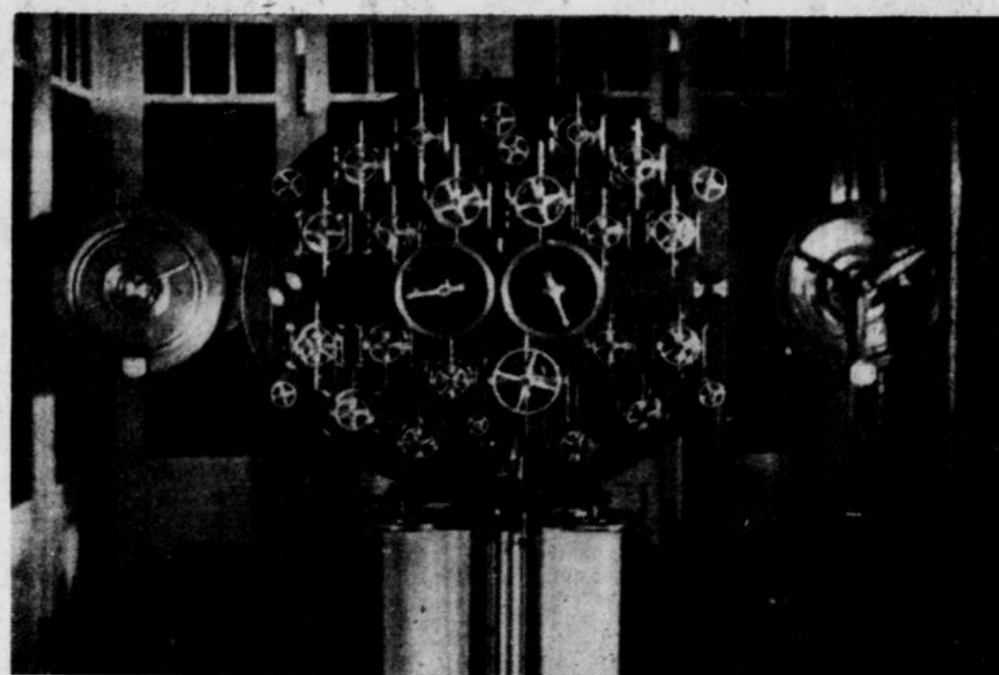
Ein Wunderwerk deutscher Feinmechanik. Die Gezeitenrechnemaschine der Seewarte Hamburg. Mit dieser Maschine ist es möglich, für viele Jahre im Voraus die Gezeiten zu berechnen. Mit der Maschine wird sozusagen der „Gezeitenfahrplan“ aufgestellt.
