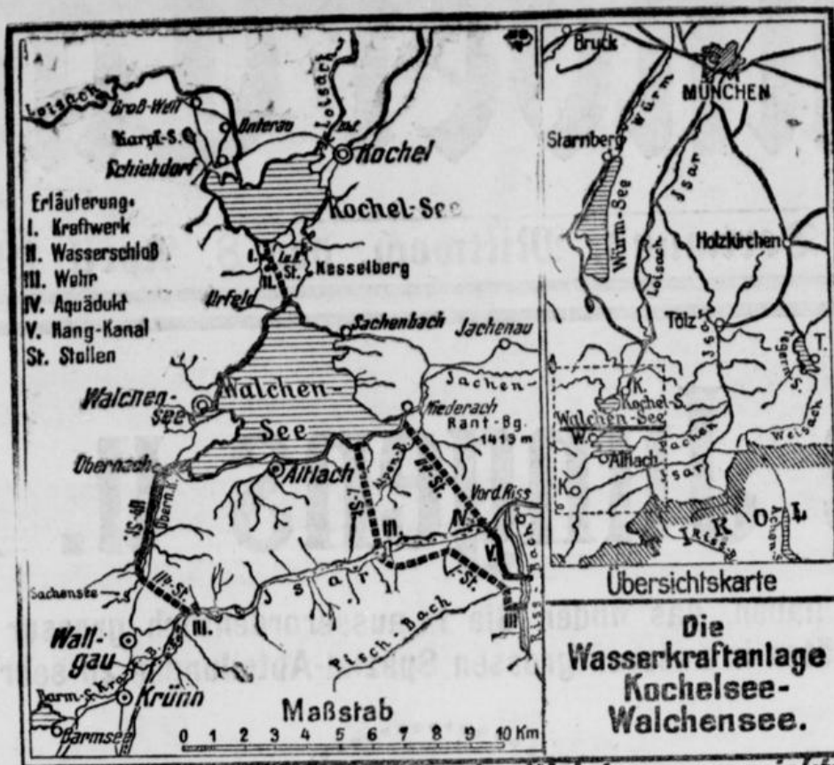
Zum bevorstehenden Ausbau des Walchenseeprojekts.
