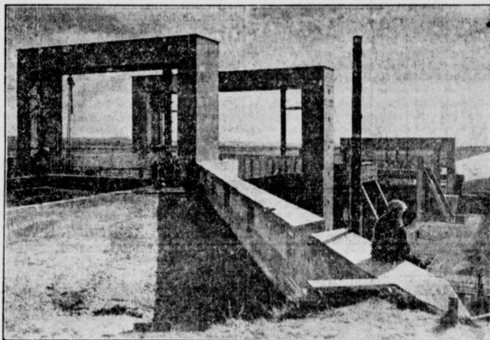
Das Schiffshebewerk Rothensee am Mittellandkanal.
