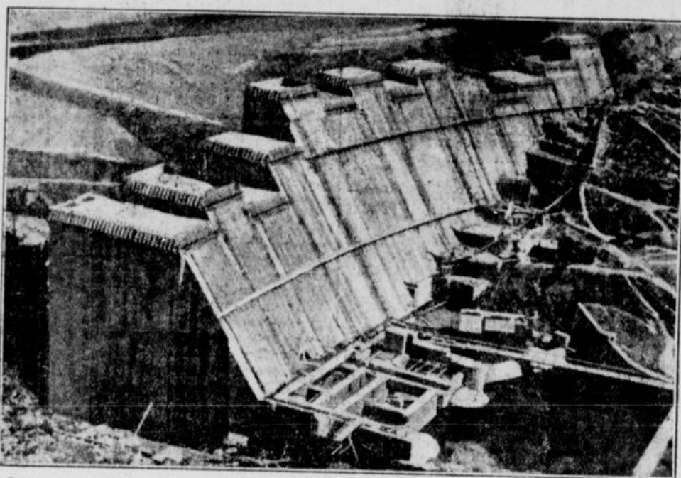
In Thüringen geht der Bau der Hohenwarthe-Talsperre rüstig vorwärts. Der größte Teil der Sperrmauer, die eine Höhe von 75 Meter erreichen und die größte Europas sein wird, ist nahezu fertig. Unser Bild vermittelt einen Eindruck von der Wucht dieses Betonriegels, der in das Flutthal (Scherl-Bilderdienst-M.)
