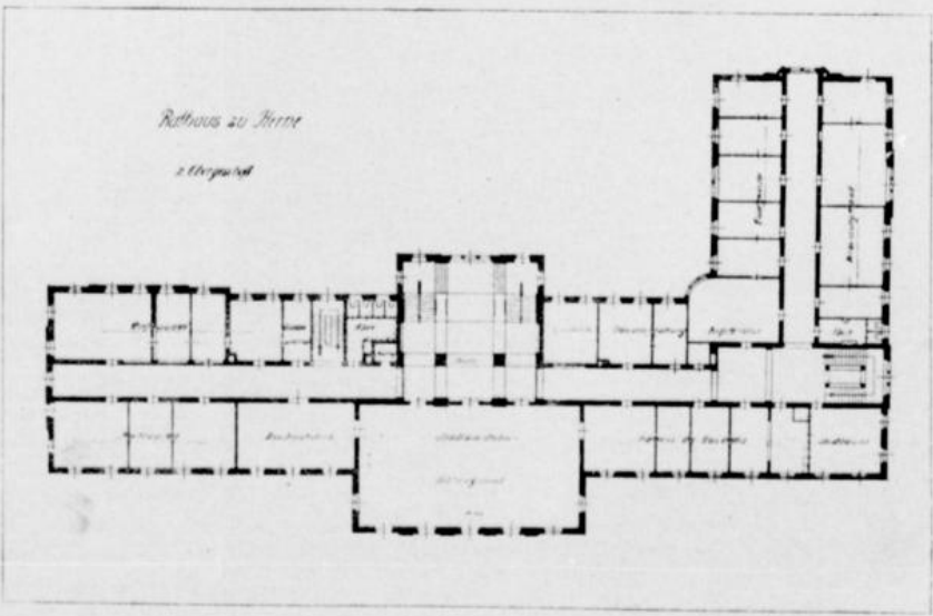
Grundriß des 2. Obergeschosses.
