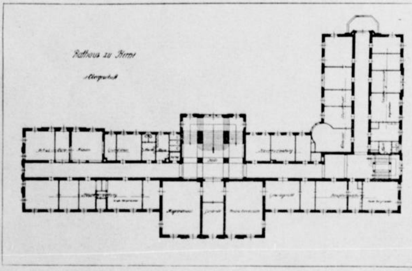
Grundriß des 1. Obergeschosses.
