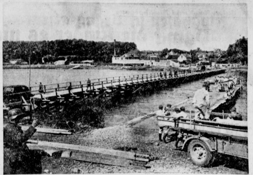
Die feste Brücke über die Loire ist fertig. Die behelfsmäßige Brücke wird von den Pionieren abgebrochen. (PK-Weber (Scherl)).
