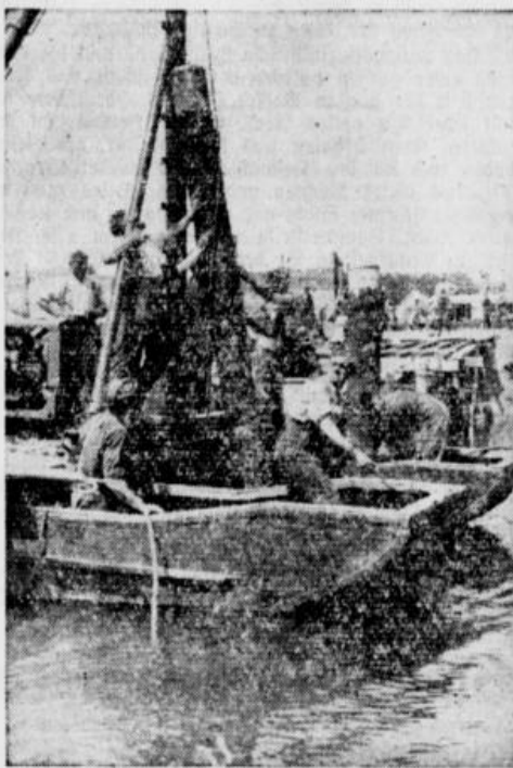
Die Verkehrswege müssen wieder hergestellt werden. Unser Bild zeigt Pioniere, die mit der Ramme Baumstämme als Pfähle in den Flußgrund rammen, um eine neue stabile Behelfsbrücke herzustellen. (PK-Fink (Scherl)).
