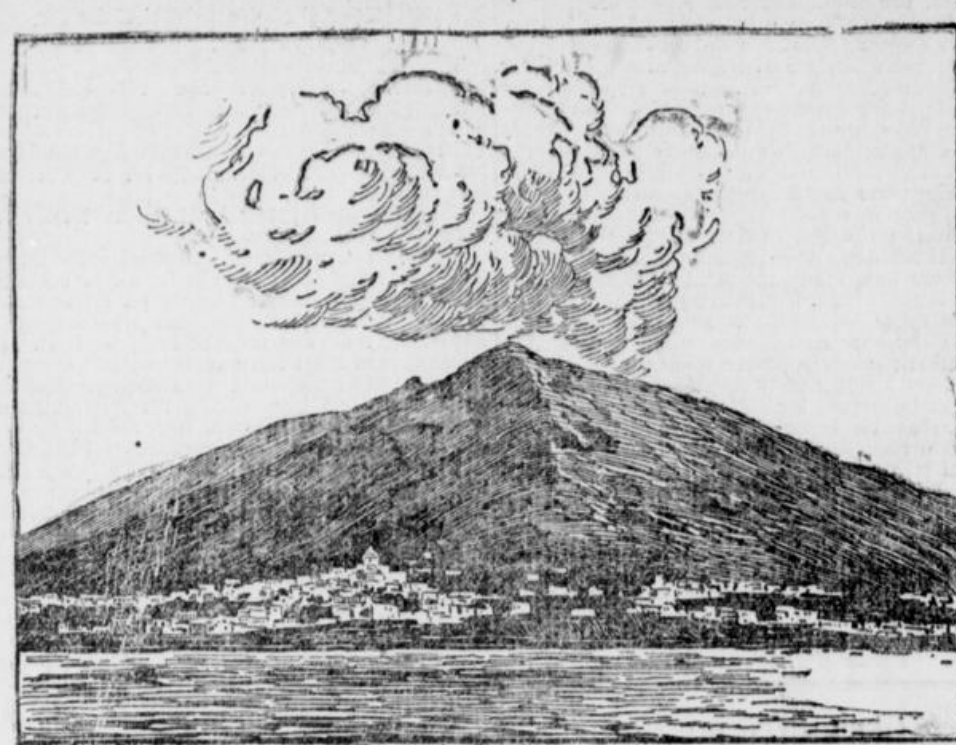
Ein neuer Ausbruch des Stromboli.
